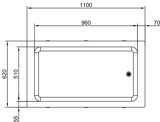
Boven aanzicht
